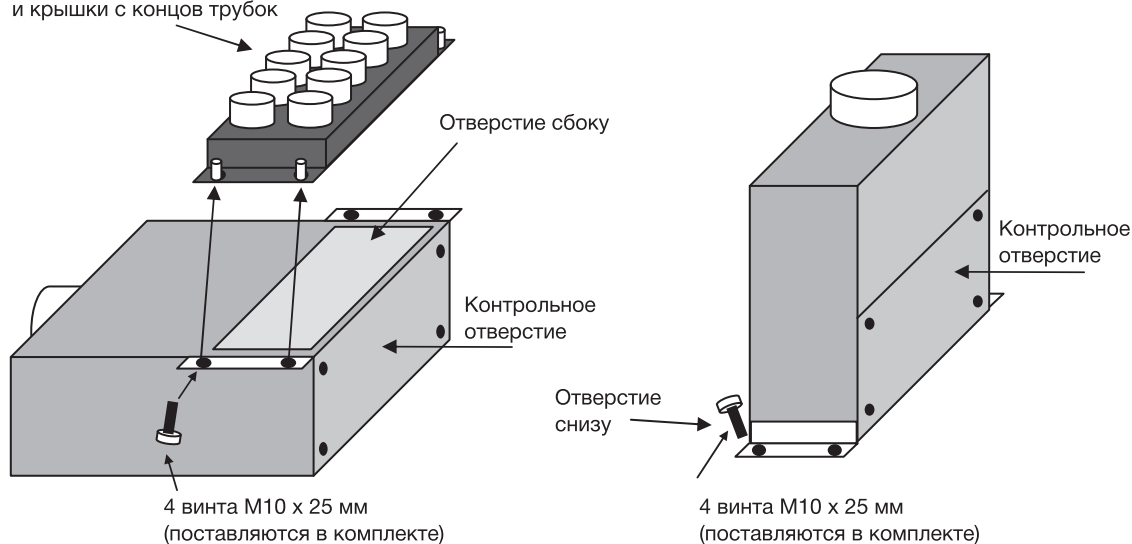
Вариант монтажа на потолке
